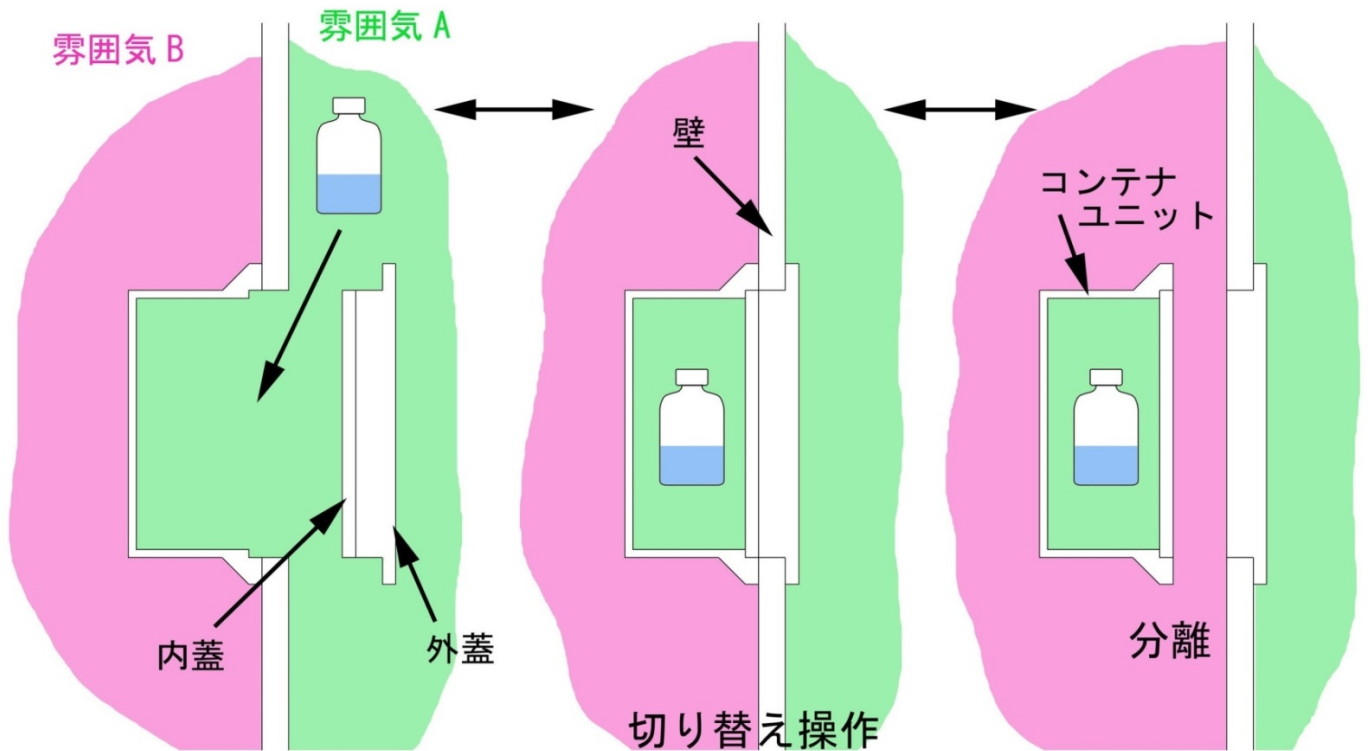
ダブルポートカバー付コンテナの概念図
